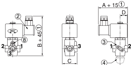
TYPE 05: NF / WSNF Aluminium; epoxy coated / AISI 316L SS EN/IEC 60079-1 and EN/IEC 60079-31
