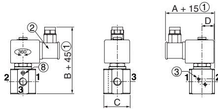
TYPE 06: NF / WSNF Aluminium; epoxy coated / AISI 316L SS EN/IEC 60079-1 and EN/IEC 60079-31
