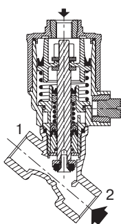
привод 32 мм
