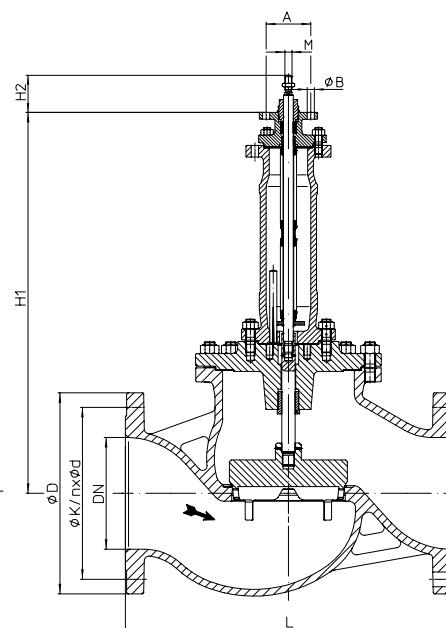
Серия 441 M16 DN200-250 (напр. PREMIO 12-25kN, AUMA SAR 07.2-10.2)
