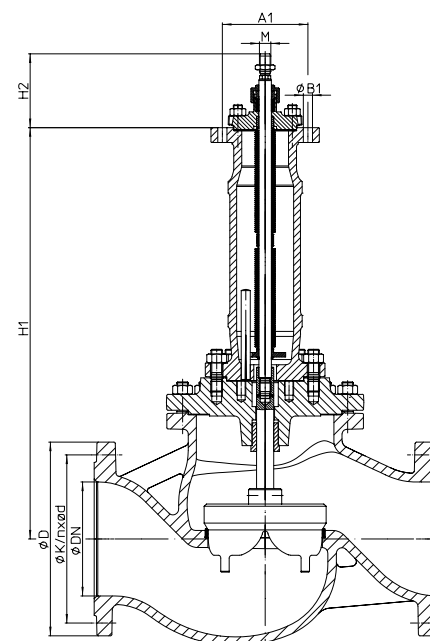
Серия 441 M20 DN200-250 (напр. DP34-34Tri)
