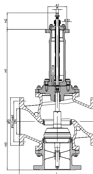
Серия 463 DN200-250 M20 (напр.: DP34-34Tri)
