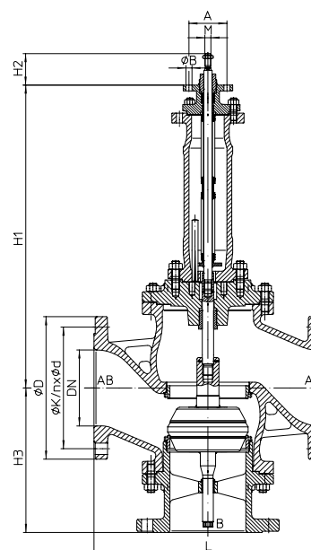
Серия 463 DN200-250 M16 (напр.: PREMIO 5-25кN; SAR 07.6 - 14.2)
