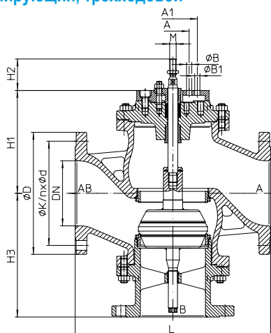
Серия 423 DN200-250 (напр.: DP34-34Tri; PREMIO 5-25кN)
