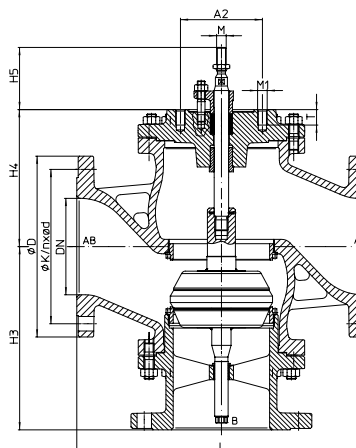
Серия 423 DN200-250 (напр.: AUMA SAR 07.6-10.2)
