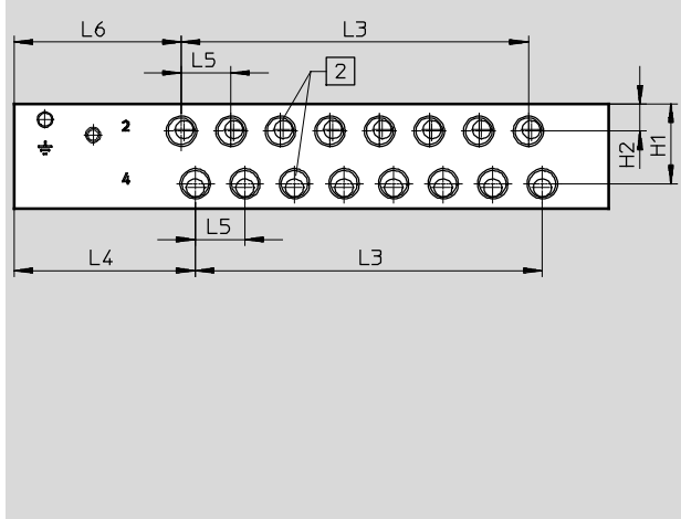
2 Канал 2/4: G1/8
