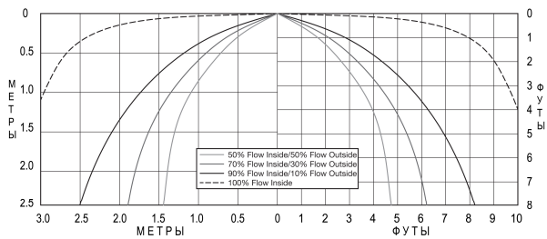
Рис. 6 Карта орошения оросителей TY325/TY323
