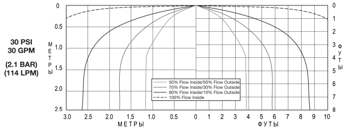
Рис. 7 Карта орошения оросителей TY315/TY313
