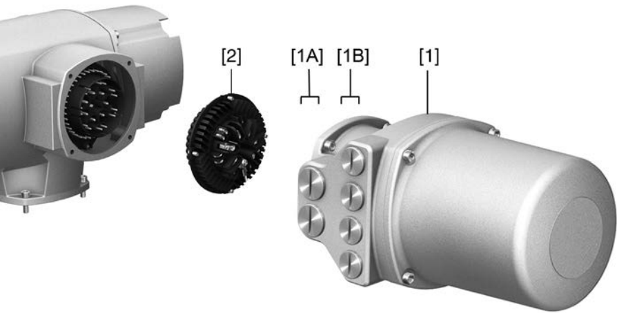
Рис.18: Электрическое подключение SFH
