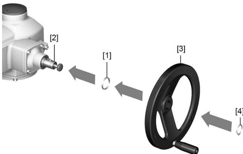
Рис.8: Маховик
