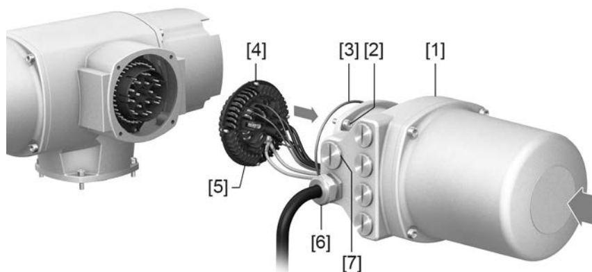
Рис.22: Порядок закрытия крышки отсека контактов двигателя для подключения к сети
