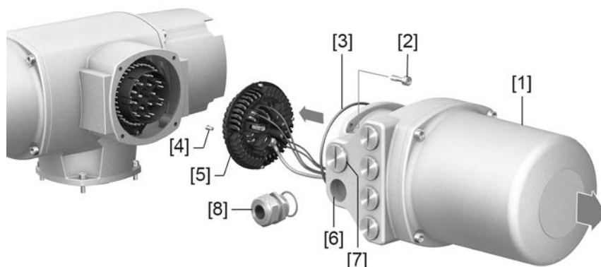
Рис.19: Откройте отсек контактов для подключения к сети
