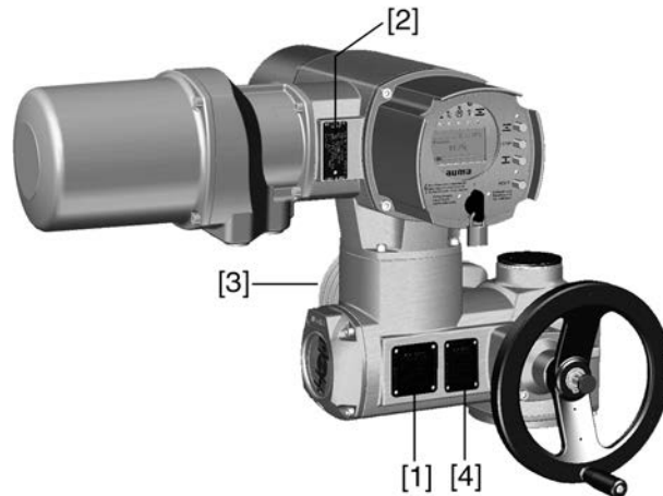
Рис.1: Вид заводской таблички
