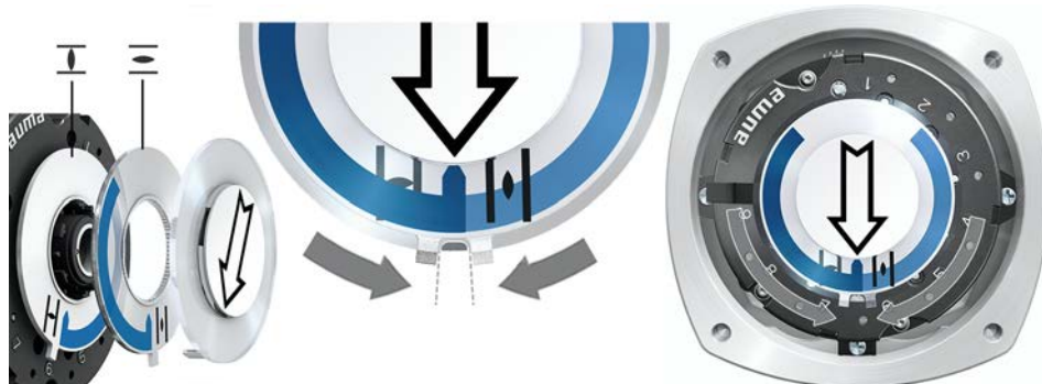
Рис.70: Позиция для настройки в положении ЗАКРЫТО
