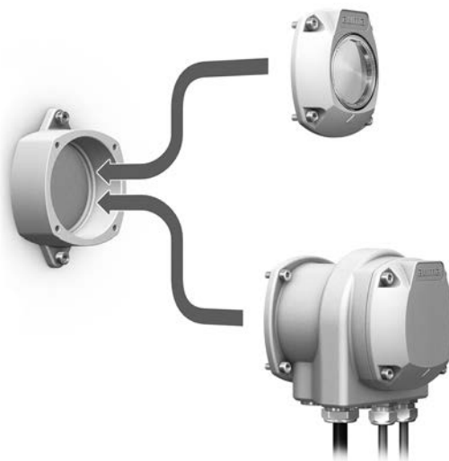
Рис.28: Защитная рамка, пример для штекера SD и крышки
