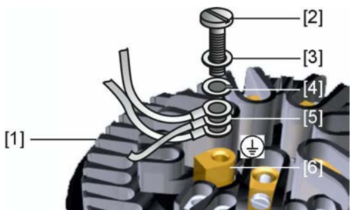
Рис.21: Разъем заземления
