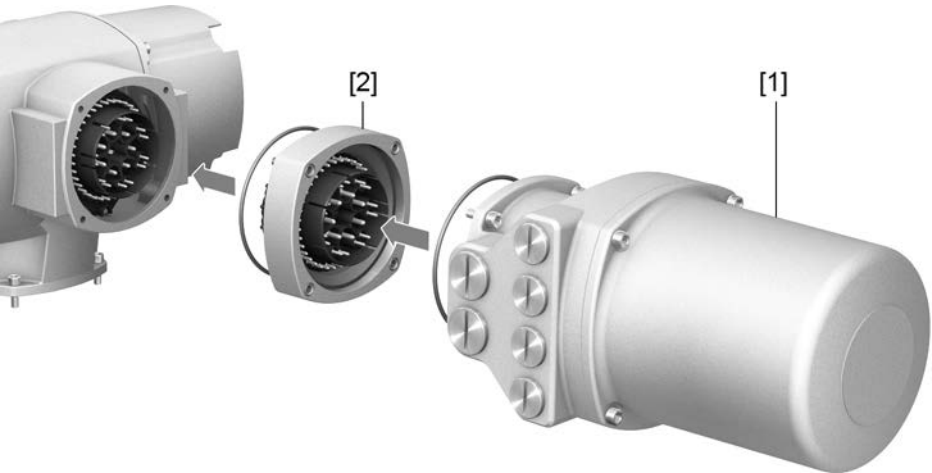
Рис.29: Электрическое подключение с промежуточной рамкой
