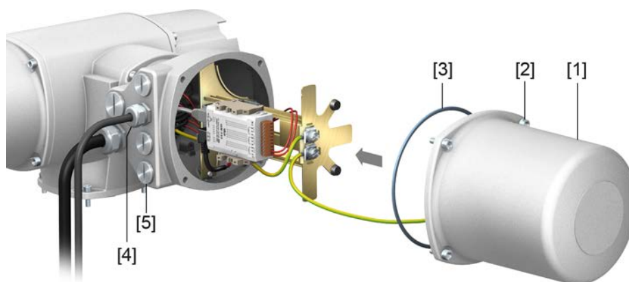
Рис.26: Закрытие разъема полевой шины
