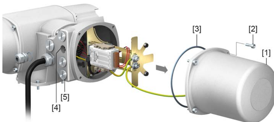
Рис.23: Открытие крышки разъема полевой шины
