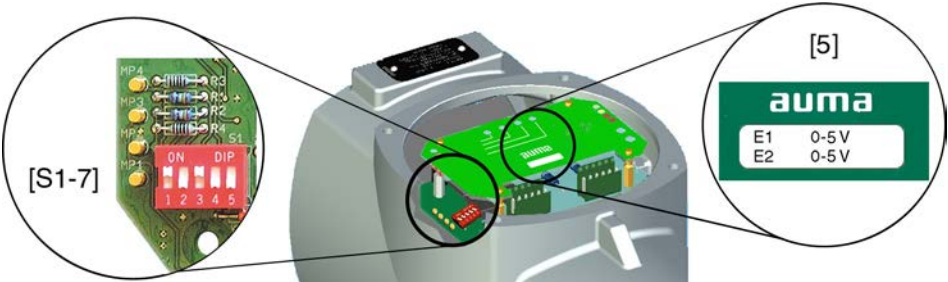
рис. 46: Исполнение с дополнительным переключателем на плате позиционера
