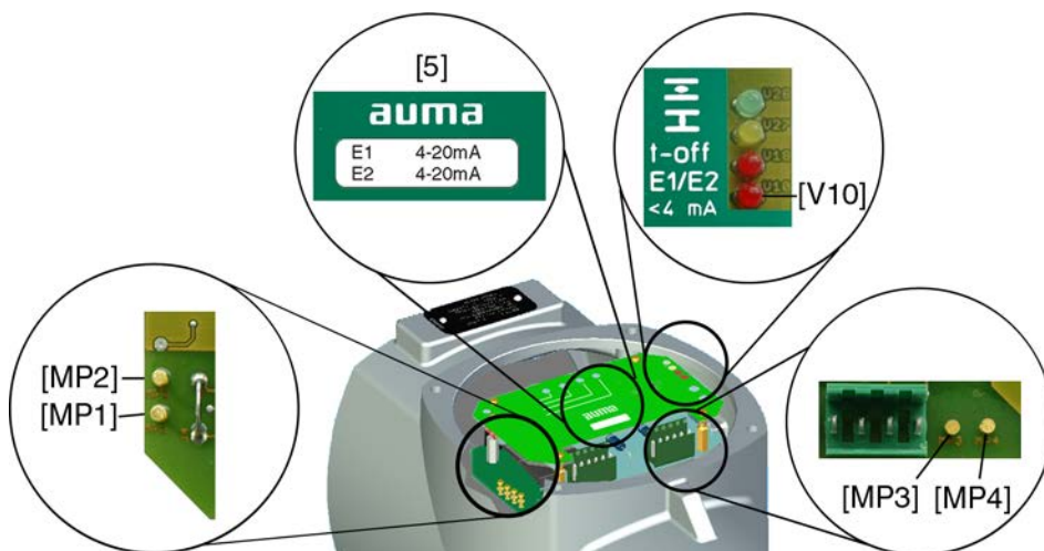
рис. 48: Плата позиционера
