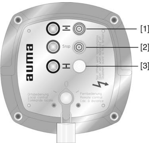
рис. 30: Панель управления с сигнальными лампами
