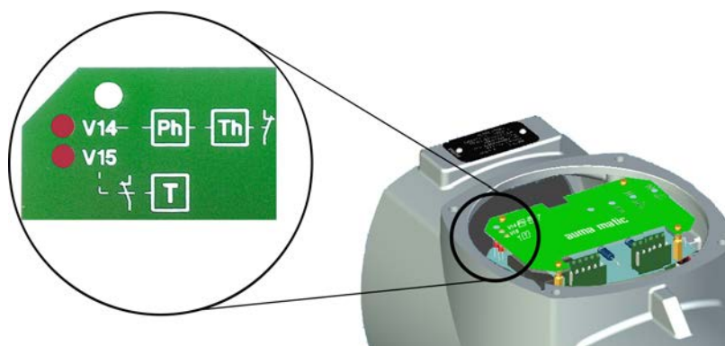
рис. 45: Индикаторы на интерфейсной плате
