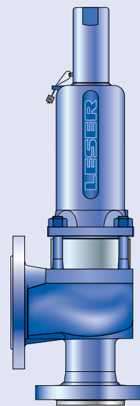
Тип 441 со сплошным соплом Колпак H2 Закрытый кожух Конструкция с уравнивающим сифоном
