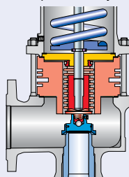
Сифон из нержавеющей стали J68: Открытый кожух J78: Закрытый кожух
