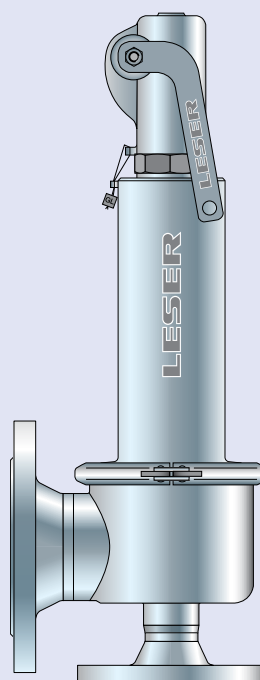
Тип 444 Герметичный рычаг H4 Закрытый кожух Стандартная конструкция
