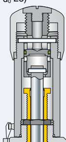
Герметичное устройство подрыва H4 Герметичная головка H4 (только d_0 \geq 23 )
