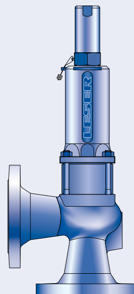
Тип 433 Колпак Н2 Закрытый кожух Конструкция с уравнивающим сифоном
