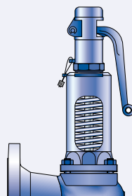
Комплект для переоборудования с установкой уравновешивающего сифона Арт. № см. стр. 02/14
