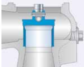
Уравновешивающий сифон J68: Открытый кожух J78: Закрытый кожух
