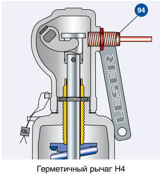
Герметичный рычаг H4
