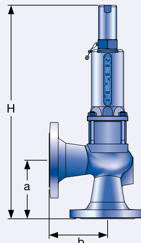
Конструкция с уравнивающим сифоном
