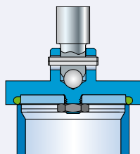
Диск с уплотнительным кольцом J20: FFKM "C" J21: CR "K" J22: EPDM "D" J23: FKM "L"
