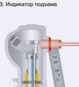
Индикатор подъема J39: Переходник H4 J93: Индикатор подъема
