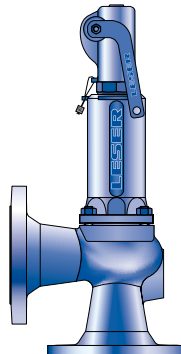
Тип 429 Герметичный рычаг Н4 Закрытый кожух Стандартная конструкция
