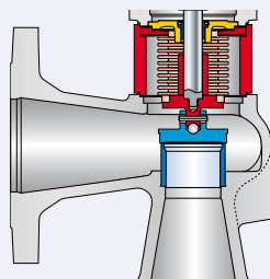
Рычаг подрыва H3 H3
