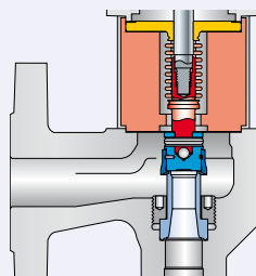
Комплект для переоборудования с установкой уравновешивающего сифона Арт. №, см. стр. 02/14
