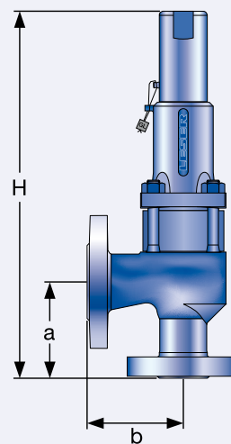
Конструкция с уравновешивающим сильфоном
