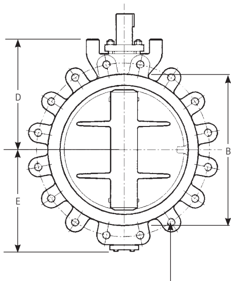
Габаритные размеры - ANSI 300
