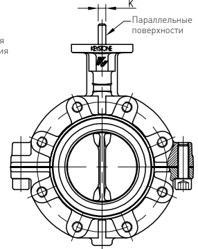
Фигура 16 с проушинами Ду 40-300
