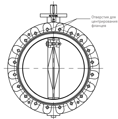
Фигура 17 с проушинами Ду 350-1000
