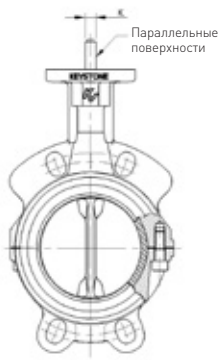
Фигура 14 вафельная Ду 40-300
