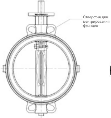
Фигура 15 вафельная Ду 350-1000
