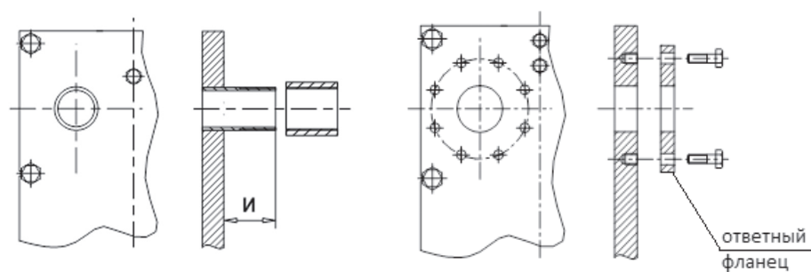
Резьбовой патрубок теплообменника
