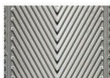
TK («мягкая») пластина
