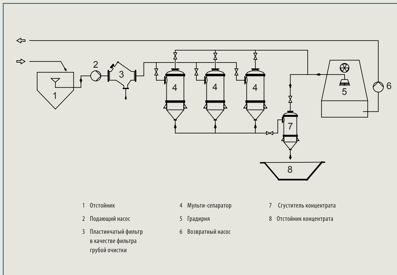
Рис. 8 Схема размещения для различных аппаратов на охлаждающем контуре ленточного стана горячей прокатки
